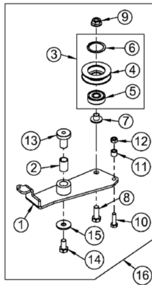
Spannrollenträger vollst.
