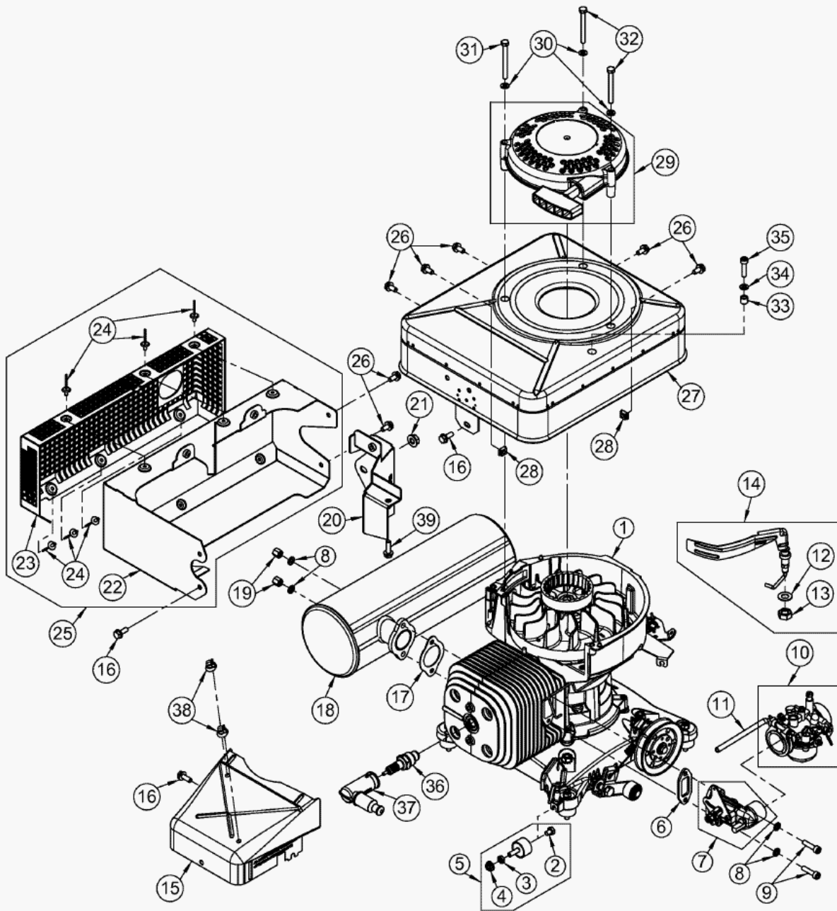
40 Antriebsblock
